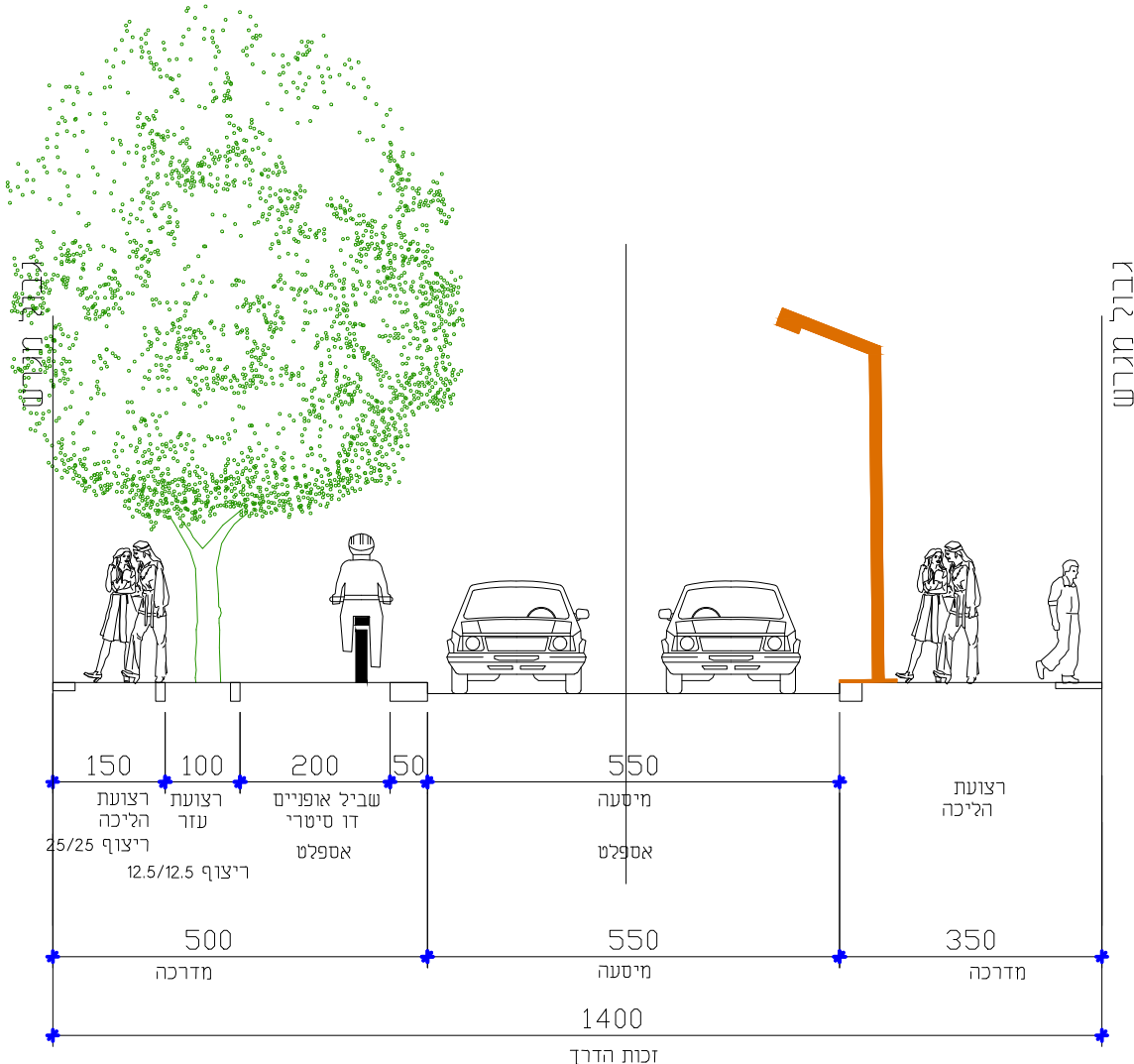
חתך ב-ב
