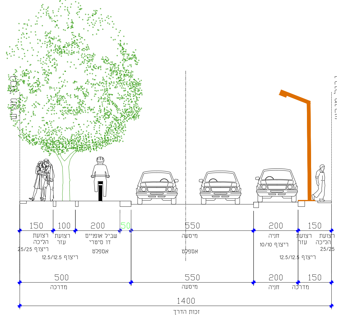
חתך א-א
