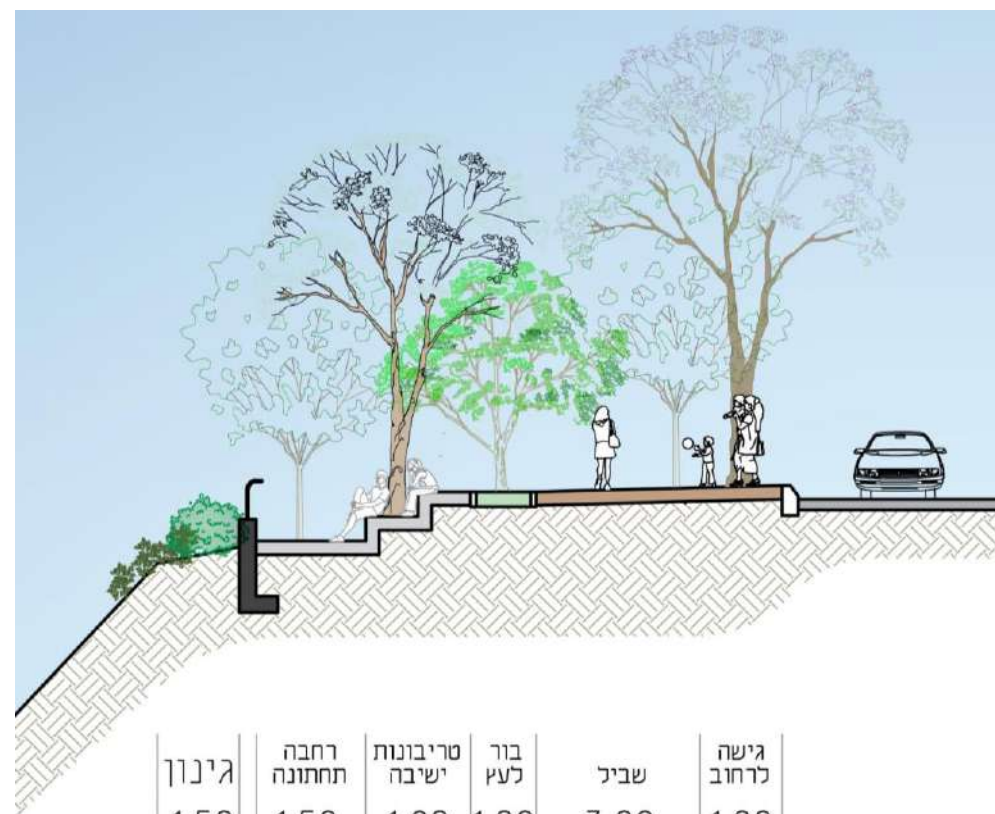
חתך ב-ב
